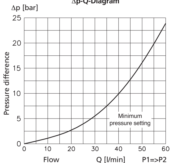
\Delta p -Q-Diagram
