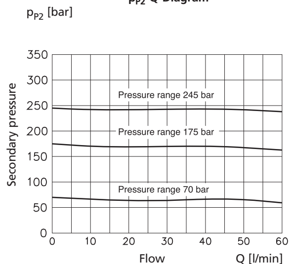
p_{P2} -Q-Diagram
